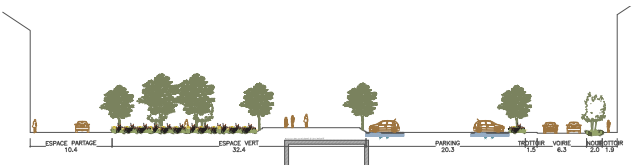
Coupe F de la proposition scénario 1 (ambition moy-
